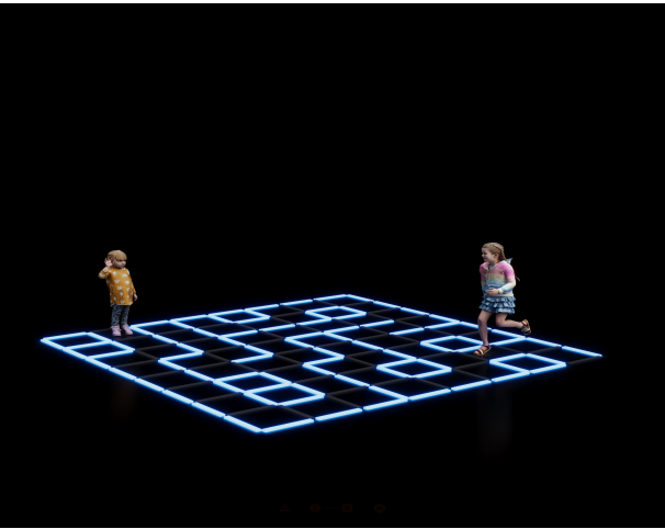
Интерактивный лабиринт
